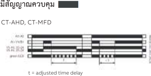
แบบสัญญาณหน่วงเวลาปิด (Signal OFF-delay) มีสัญญาณควบคุม
