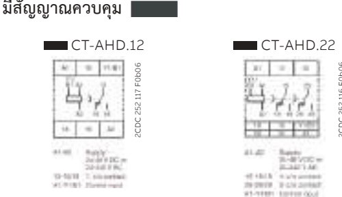
แบบสัญญาณหน่วงเวลาปิด (Signal OFF-delay) มีสัญญาณควบคุม
